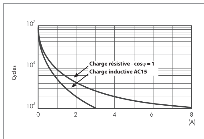
F 40.2 - Durée de vie électrique (AC) en fonction de la charge
