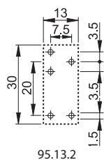
95.13.2 Vue côté cuivre
