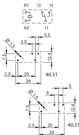
Vue coté cuivre
