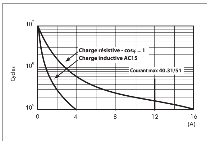
F 40.6 - Durée de vie électrique (AC) en fonction de la charge
