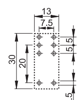
95.15.2 Vue côté cuivre
